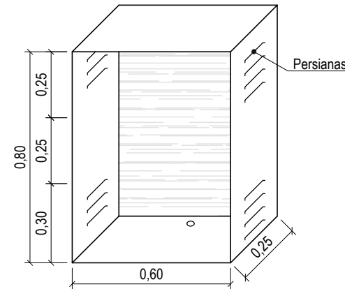
Perspectiva Escala 1 : 20
