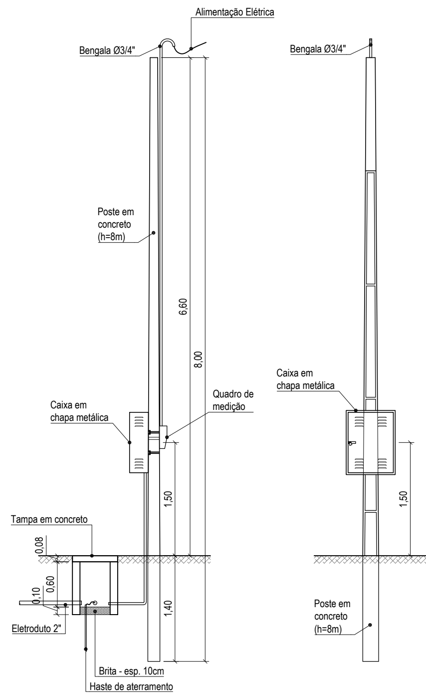
Detalhe do Poste - Vista Lateral e Frontal Escala 1 : 50
