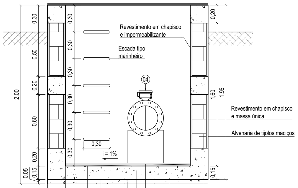
Corte B-B Escala 1 : 25
