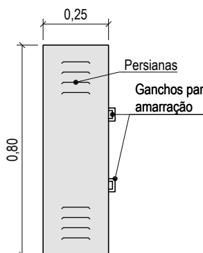
Vista Lateral Escala 1 : 20
