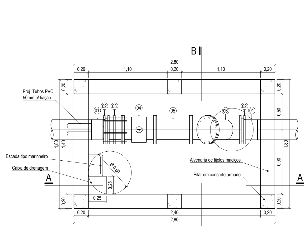
Planta Baixa Escala 1 : 25
